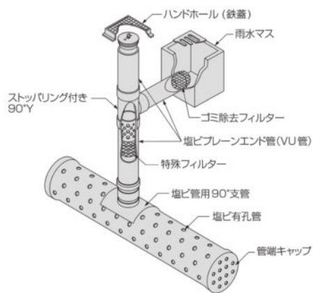
■道路排水用横型雨水浸透ユニット (SP-Hユニット)
