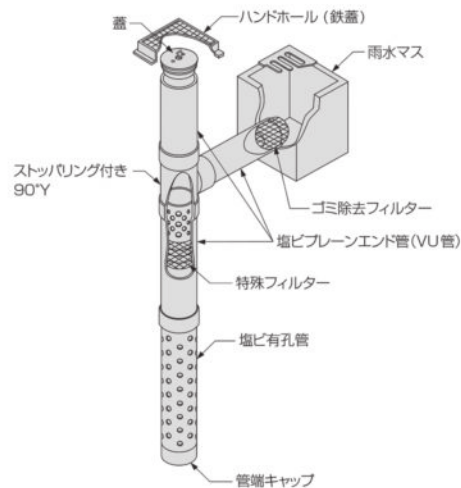
■道路排水用縦型雨水浸透ユニット (SP-Vユニット)
