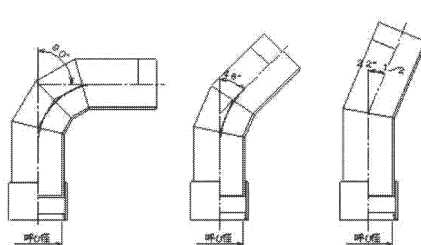
構造図
