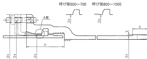
A部詳細
