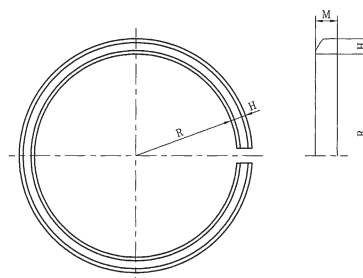
呼び径500～1000
