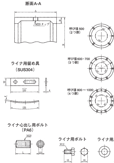
呼び径 500～1000
