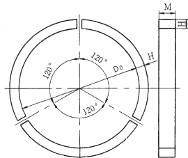
呼び径100・150
