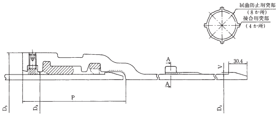
断面A-A
