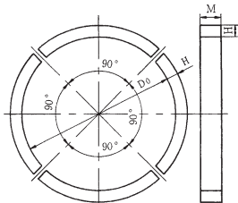
呼び径75・200・250
