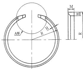
呼び径150～250
