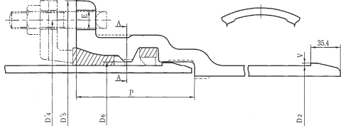
断面A-A
