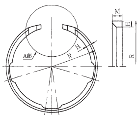
呼び径300～450
