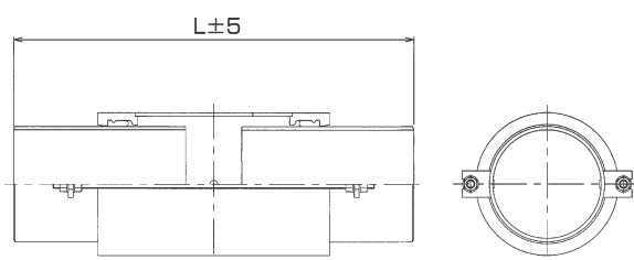
BB図面
