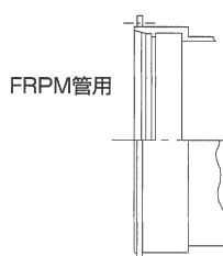
(3) 受 口(U)
