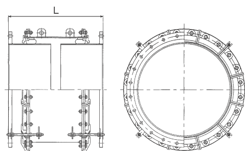
FF図面
