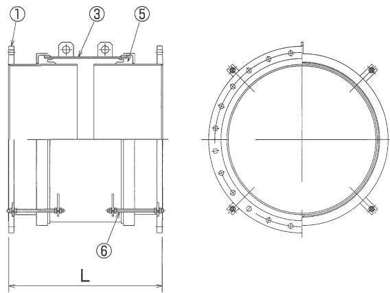
E9図面
