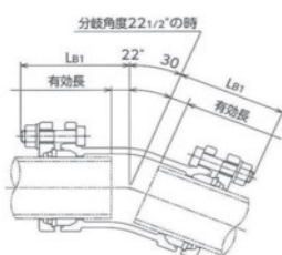
呼び径50mm NSP-GLS(曲管)
