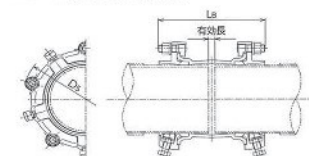
NSP-GL (離脱防止押輪付)
