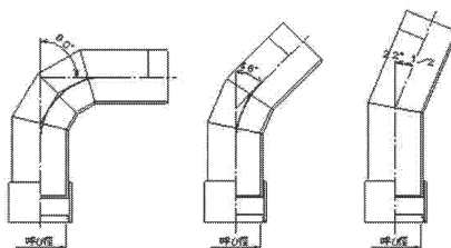
構造図
