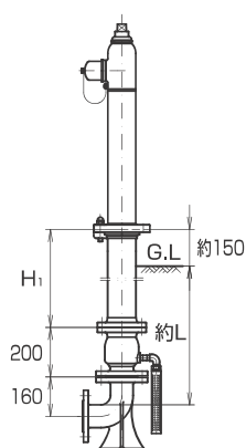
呼び径75mm Ⅱ型 回転打倒式 乙管付
