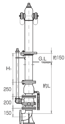
呼び径100mm Ⅱ型 回転打倒式 補修弁・乙管付
