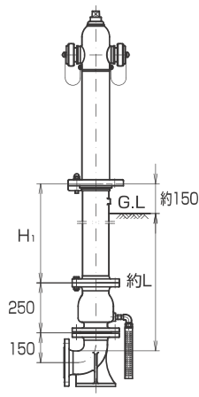
呼び径100mm Ⅱ型 回転打倒式 乙管付
