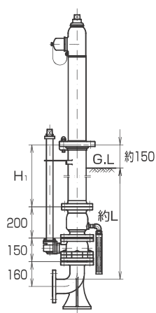
呼び径75mm Ⅱ型 回転打倒式 補修弁・乙管付
