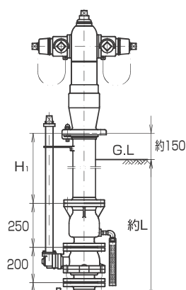
呼び径100mm 回転打倒式 補修弁・乙管付
