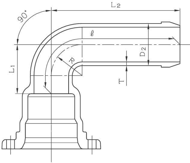
S 50 形 曲管 90°
