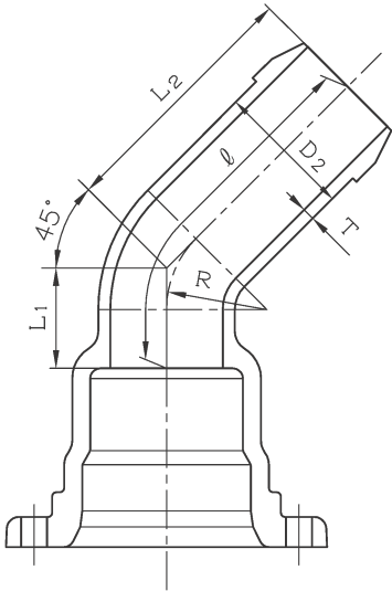
S 50 形 曲管 45°
