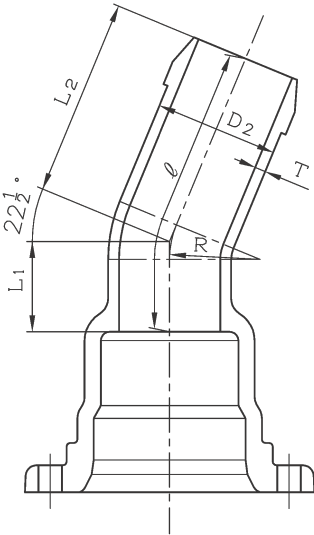
S 50 形 曲管 22 1/2°
