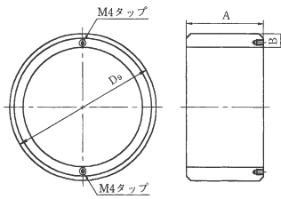
呼び径 75～250
