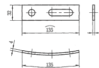
ライナ用留め具 (SUS304)
