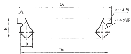
タイプⅡ 呼び径75～250直管用、異形管用
