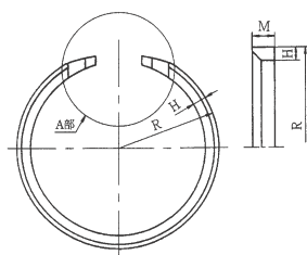
呼び径 150～250
