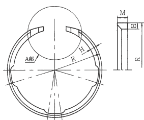
呼び径 300～450
