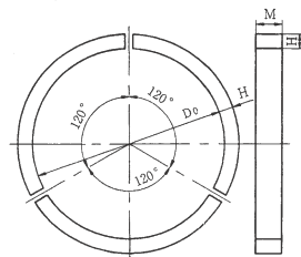
呼び径 100・150
