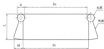
呼び径500～1000直管用及び異形管用
