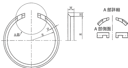
呼び径 300～450
