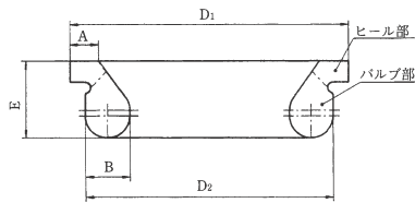
タイプⅠ 呼び径300～450直管用
