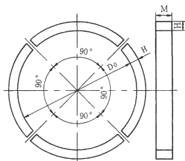
呼び径 75・200・250
