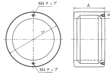
各部寸法の許容差
