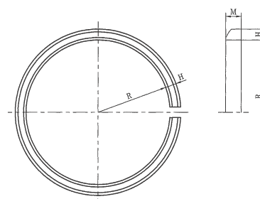
呼び径 500～1000
