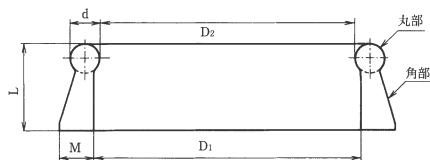
呼び径75～250継ぎ輪用、帽用及び呼び径300～450異形管用
