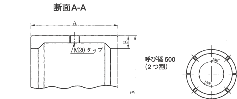
呼び径 500～1000
