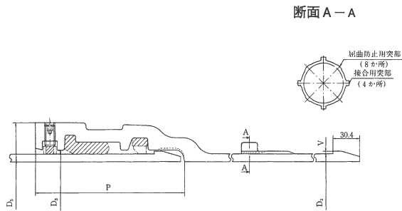
NS形 ダクタイル鋳鉄異形管 (1) 呼び径75~250
